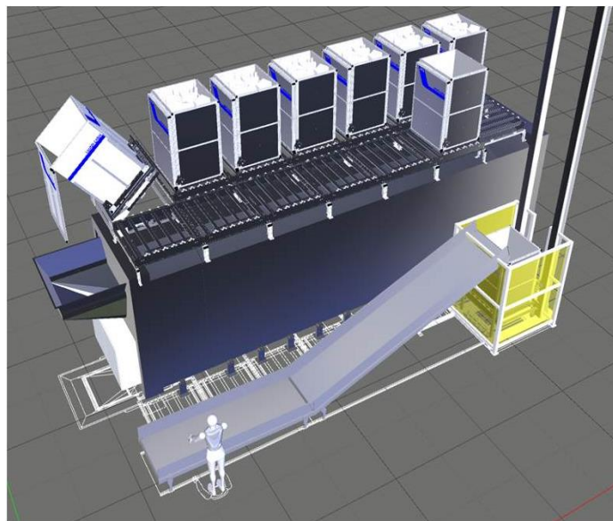
最小の作業員での生産プロセスイメージ図
