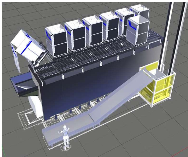
最小の作業員での生産プロセスイメージ図
